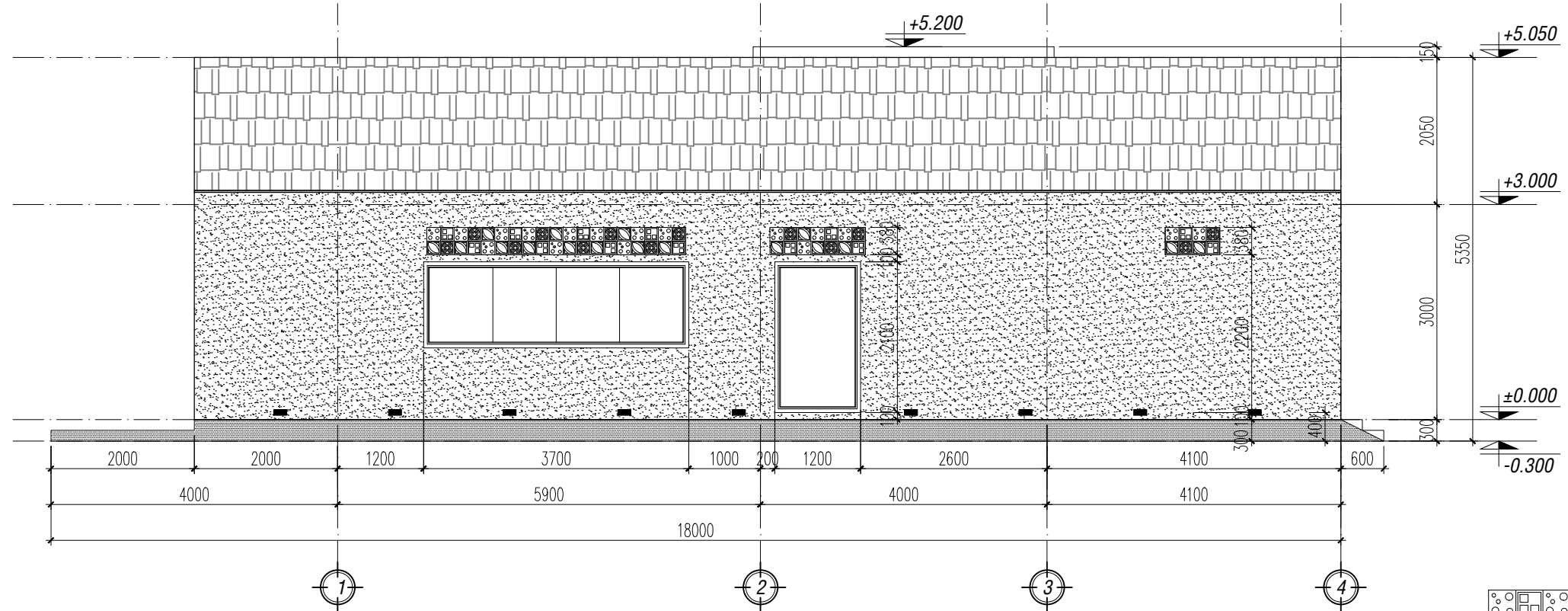
RIGHT ELEVATION
